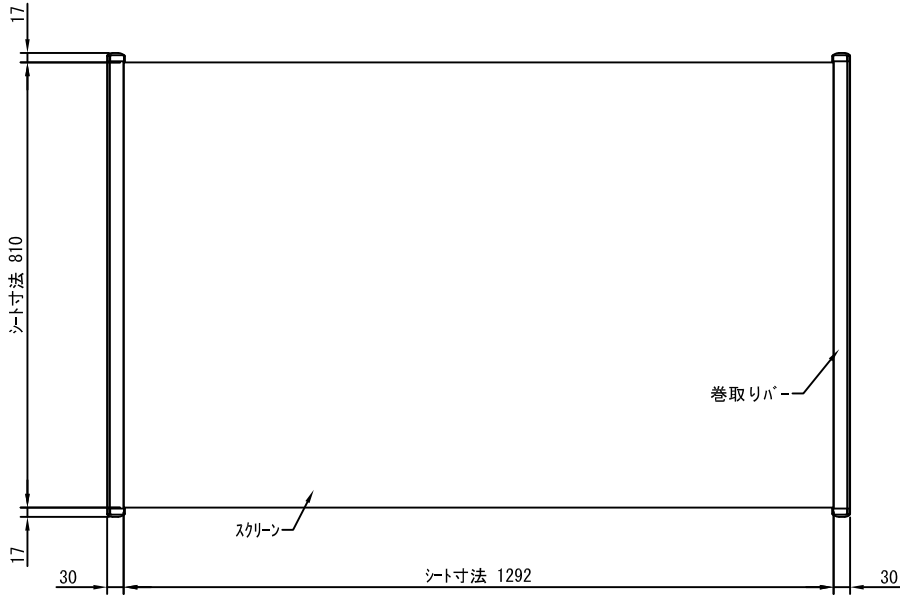
外観図 1/30
