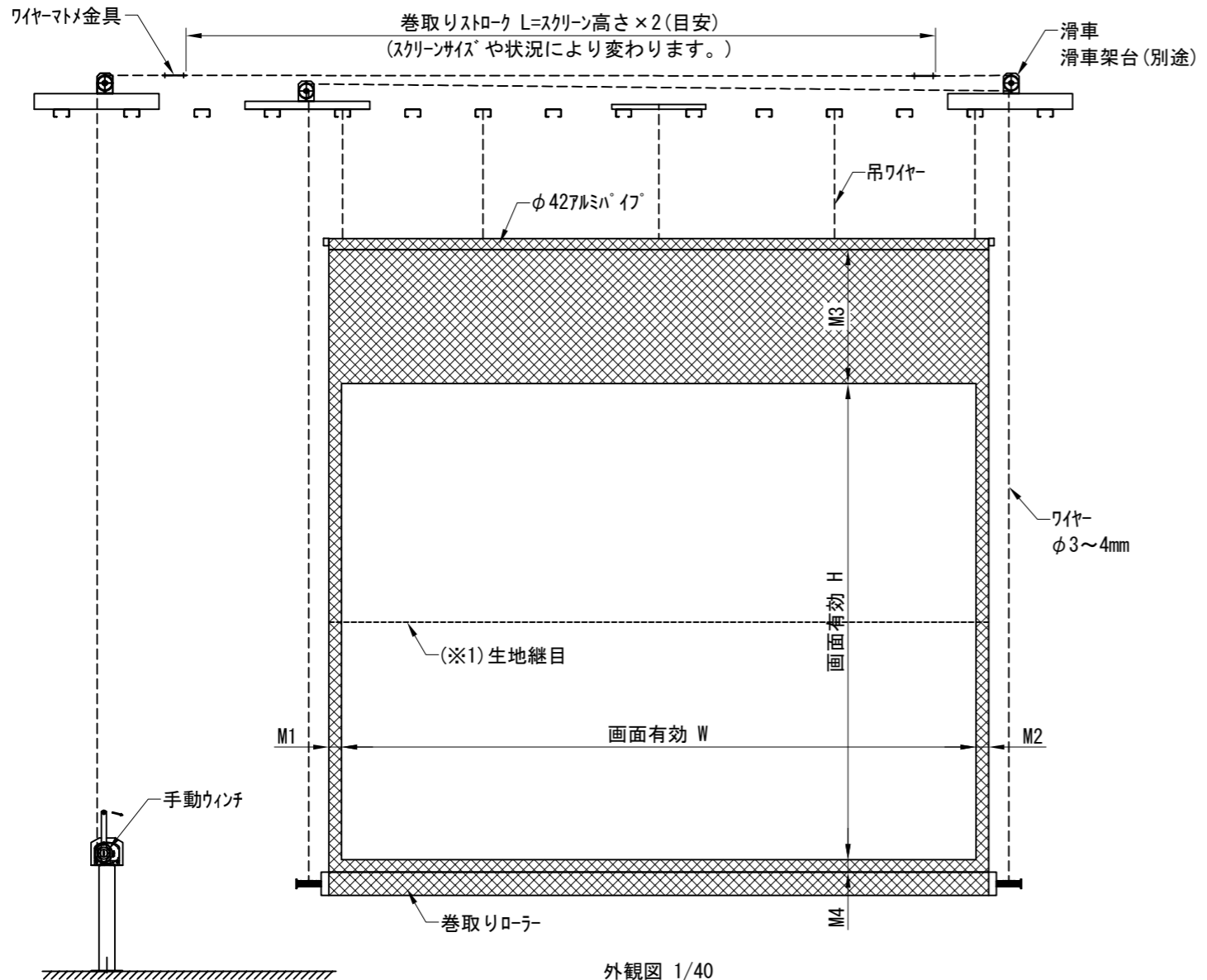
外観図 1/40
