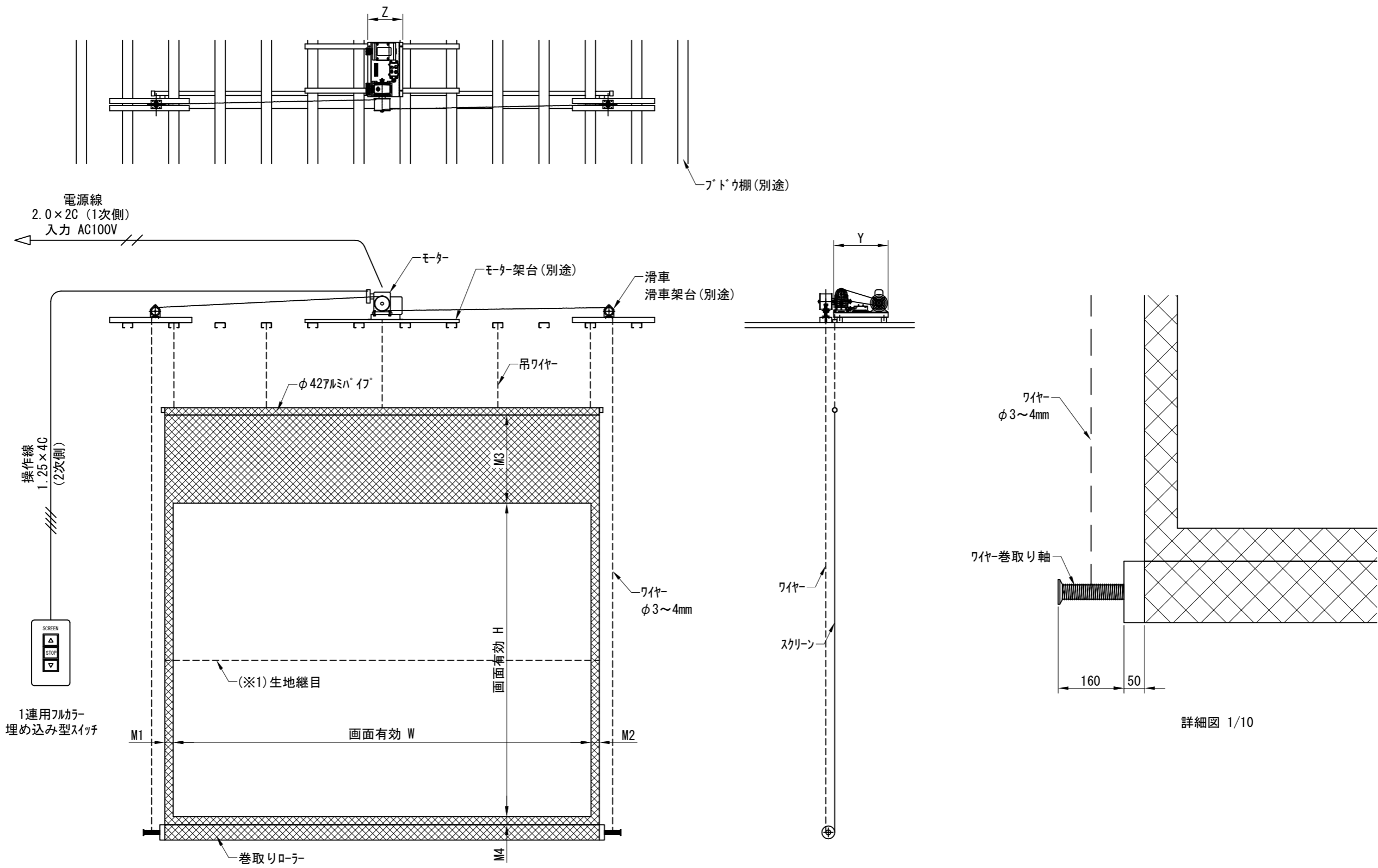
外観図 1/40
