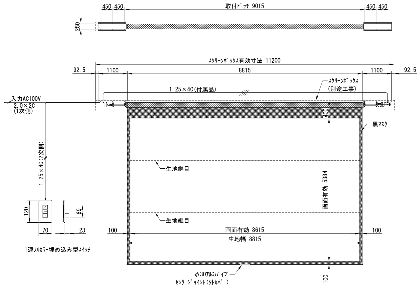
外観図 1/70
