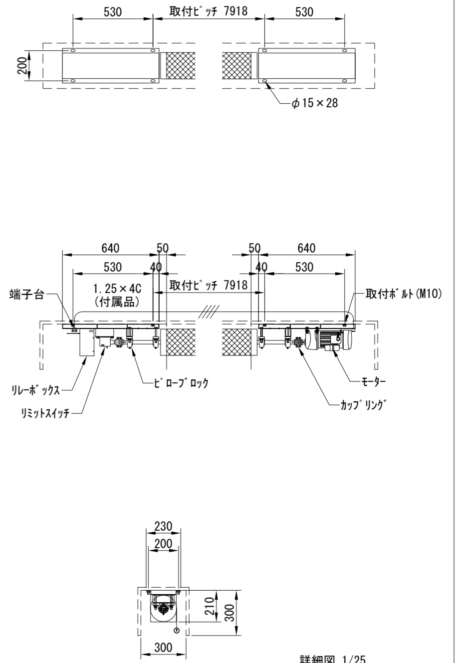
詳細図 1/25
