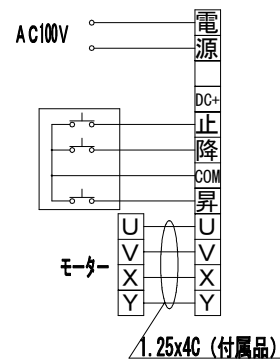
結線図
