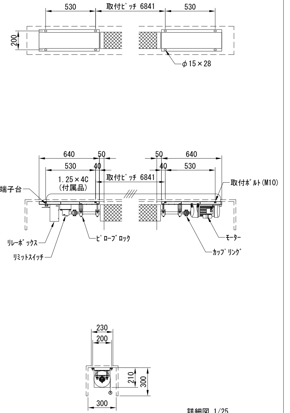
詳細図 1/25
