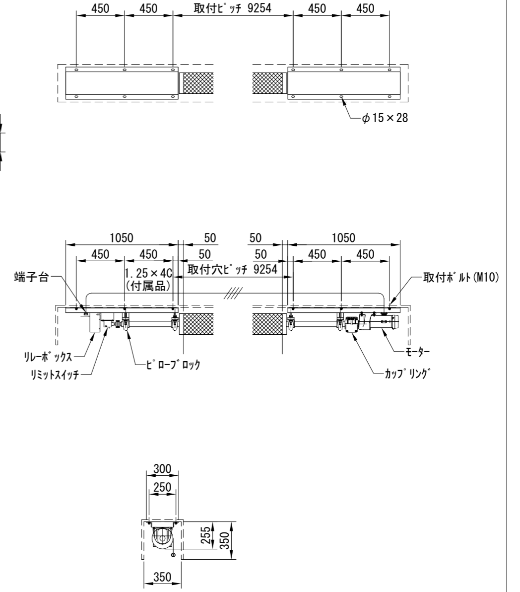
詳細図 1/35
