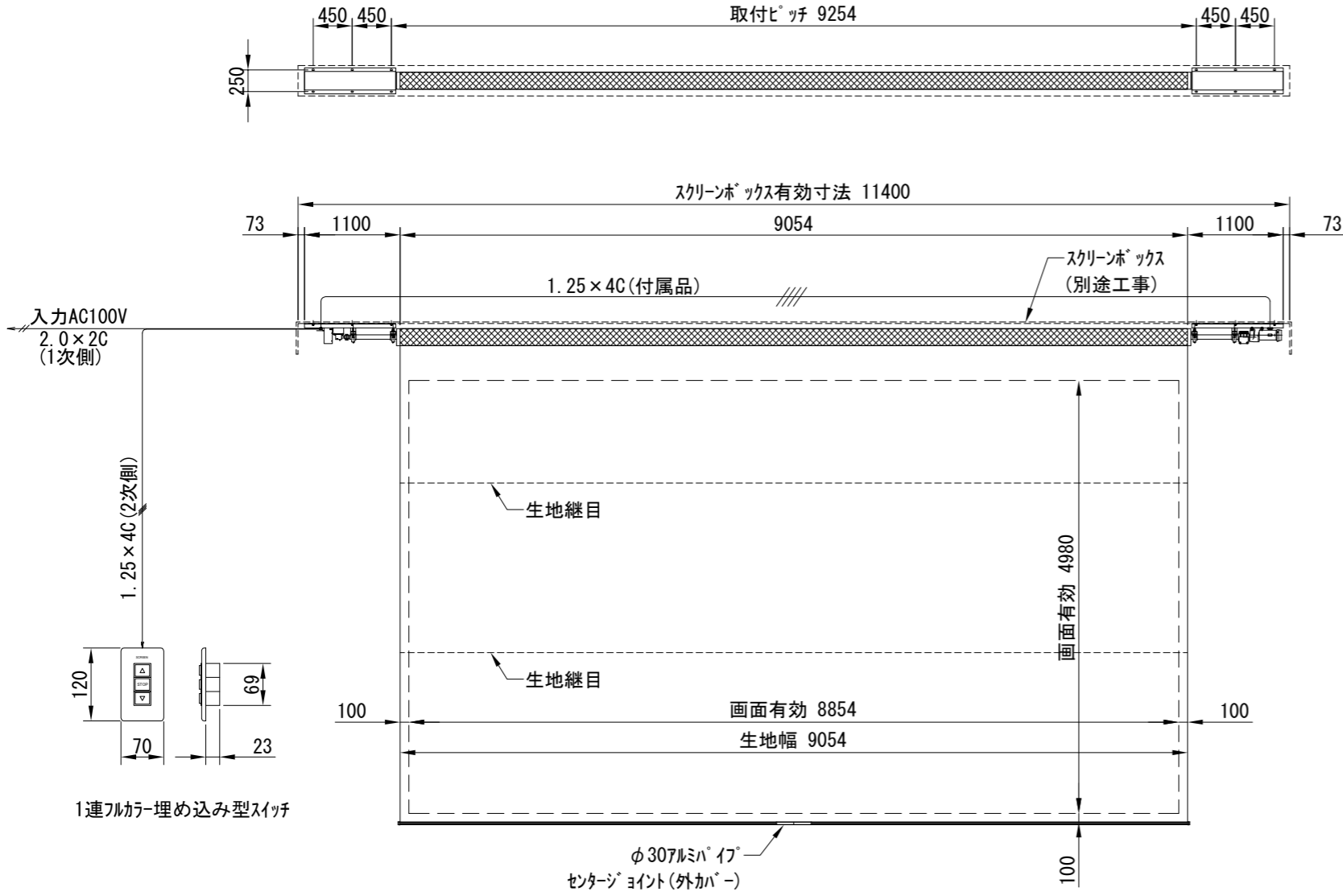
外観図 1/70
