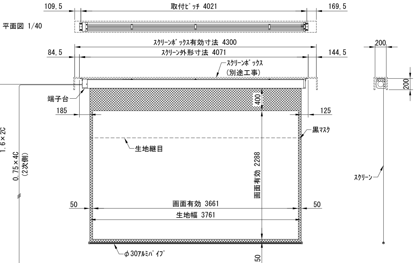
外観図 1/40
